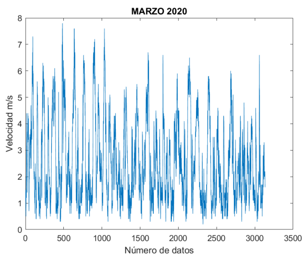
Figura 95. Velocidad del viento 03/2020.
