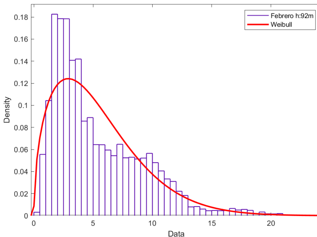
Figura 137. Distribución de Weibull mes febrero H: 92 metros.
