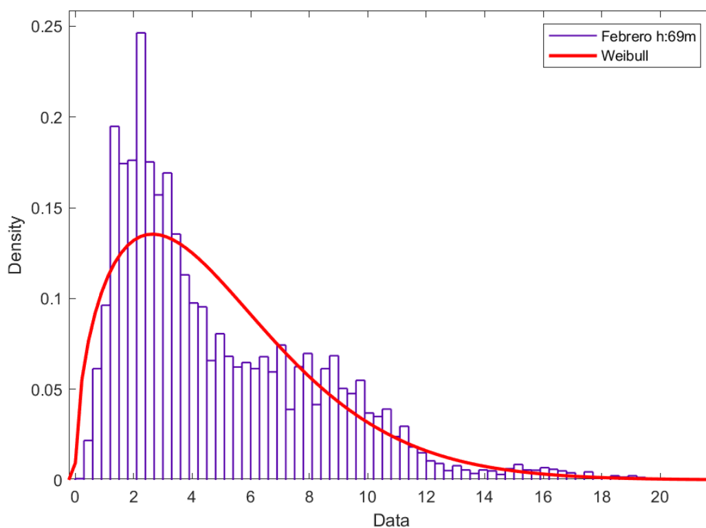
Figura 111. Distribución de Weibull mes febrero H: 69 metros.
