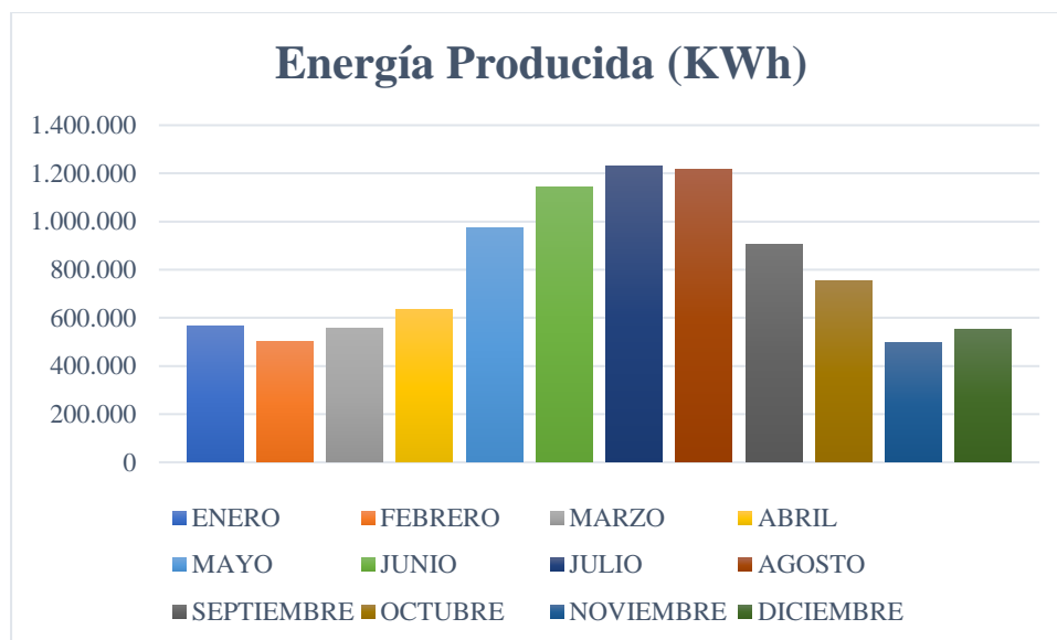
Figura 157. Energía producida mensual por el aerogenerador Alstom ECO 122/2700.
