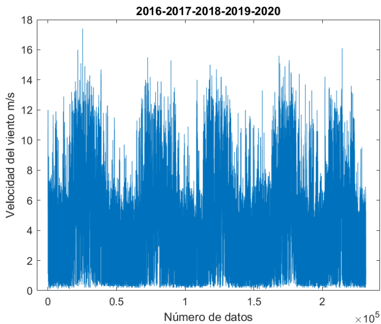
Figura 44. Velocidades del viento finales.
