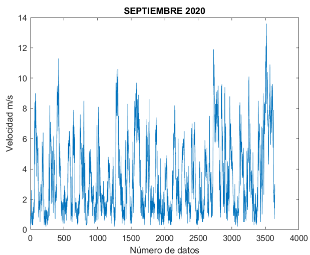
Figura 101. Velocidad del viento 09/2020.
