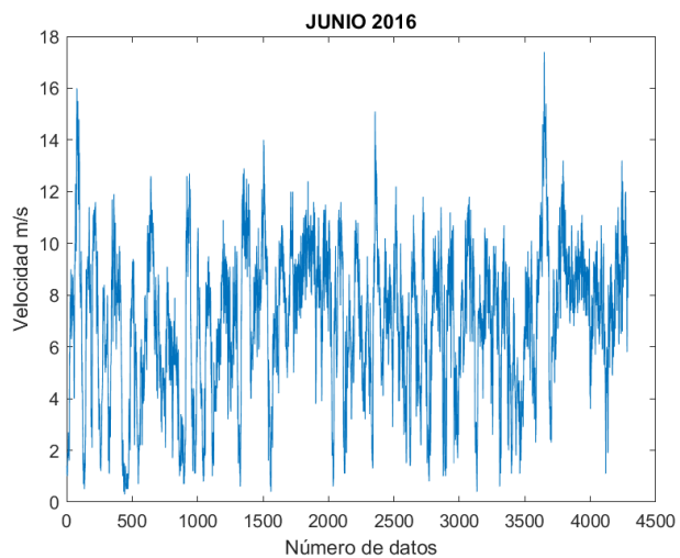
Figura 50. Velocidad del viento 06/2016.
