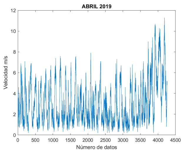
Figura 84. Velocidad del viento 04/2019.
