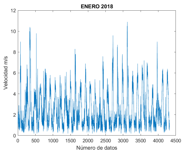
Figura 69. Velocidad del viento 01/2018.
