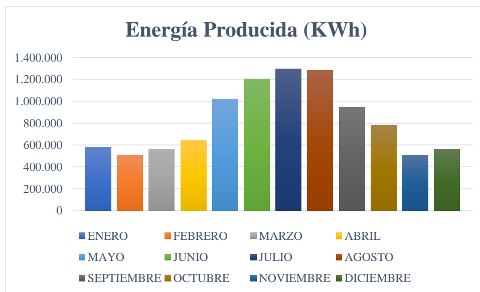
Figura 158. Energía producida aerogenerador Enercon E115/3000.
