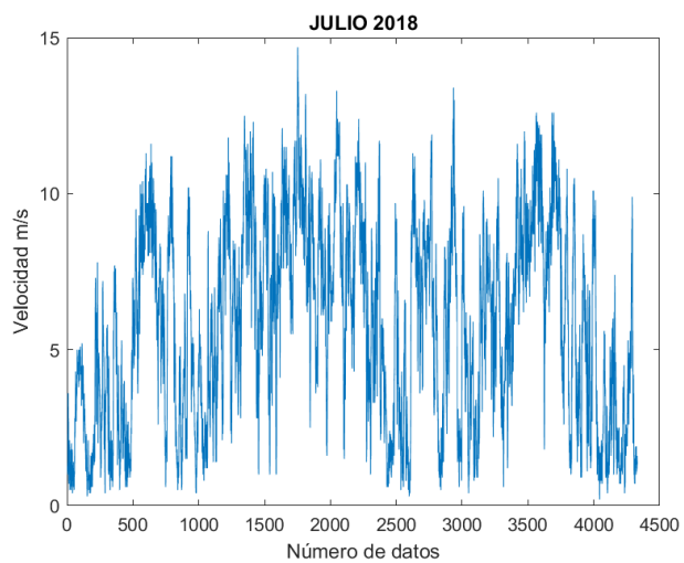
Figura 75. Velocidad del viento 07/2018.
