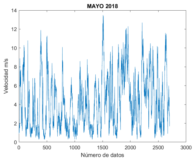
Figura 73. Velocidad del viento 05/2018.
