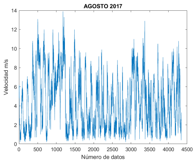
Figura 64. Velocidad del viento 08/2017.
