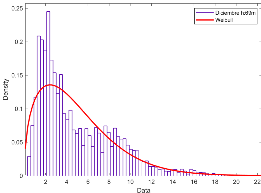
Figura 121. Distribución de Weibull mes diciembre H: 69 metros.
