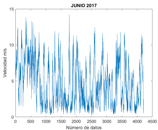
Figura 62. Velocidad del viento 06/2017.
