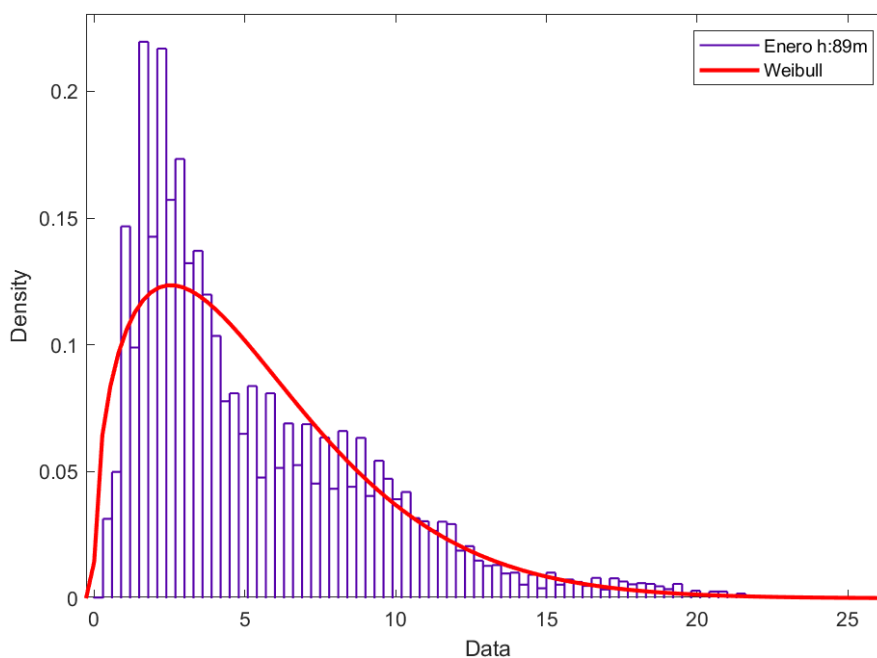
Figura 123. Distribución de Weibull mes enero H: 89 metros.
