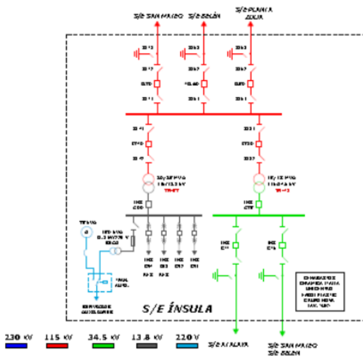
Figura 179. Diagrama unifilar subestación eléctrica Ínsula. Tomado de: CENS.
