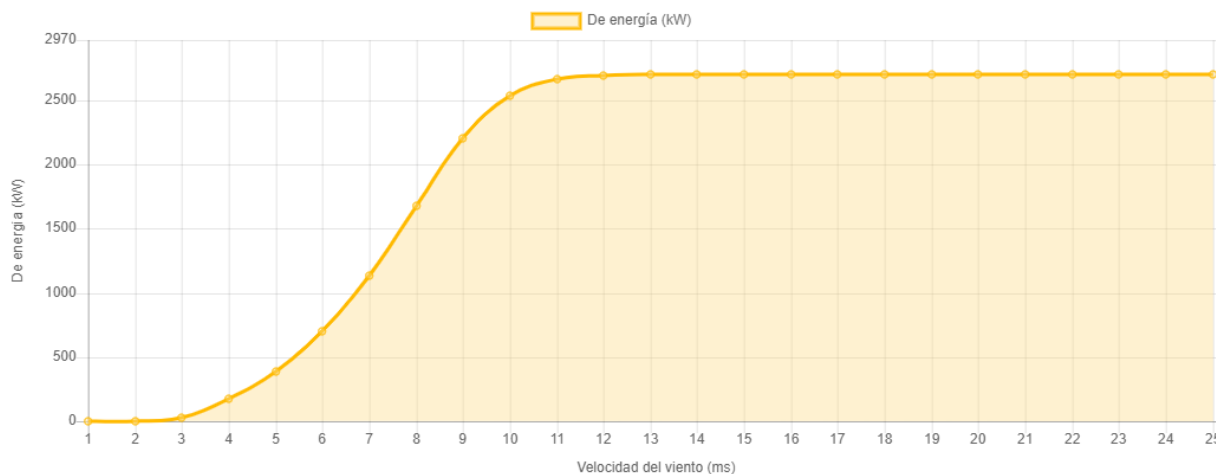
Figura 153. Curva de potencia aerogenerador Alstom ECO 122/2700. Tomado de: (wind-turbine-models.com, 2022)
