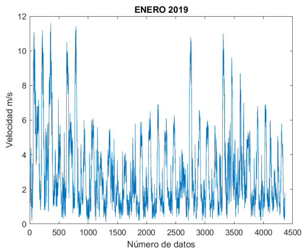
Figura 81. Velocidad del viento 01/2019.
