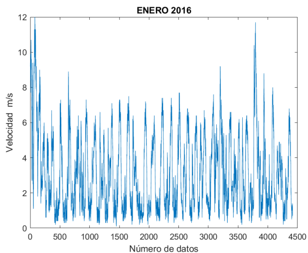
Figura 45. Velocidad del viento 01/2016.
