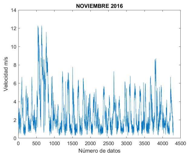
Figura 55. Velocidad del viento 11/2016.
