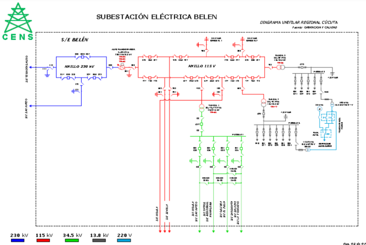
Figura 175. Diagrama unifilar subestación eléctrica Belén. Tomado de: CENS.
