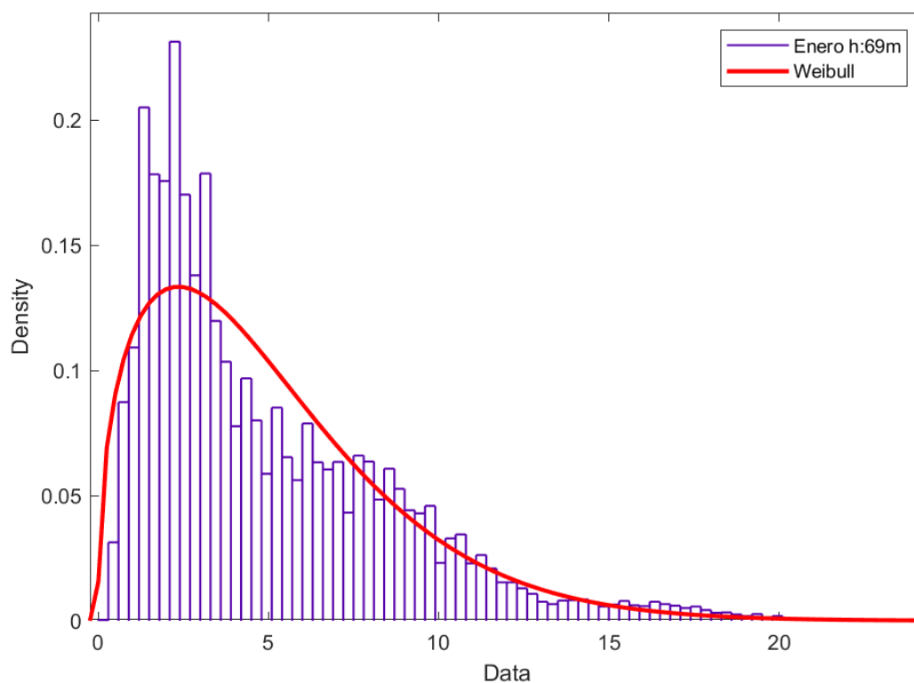
Figura 110. Distribución de Weibull mes enero H: 69 metros.
