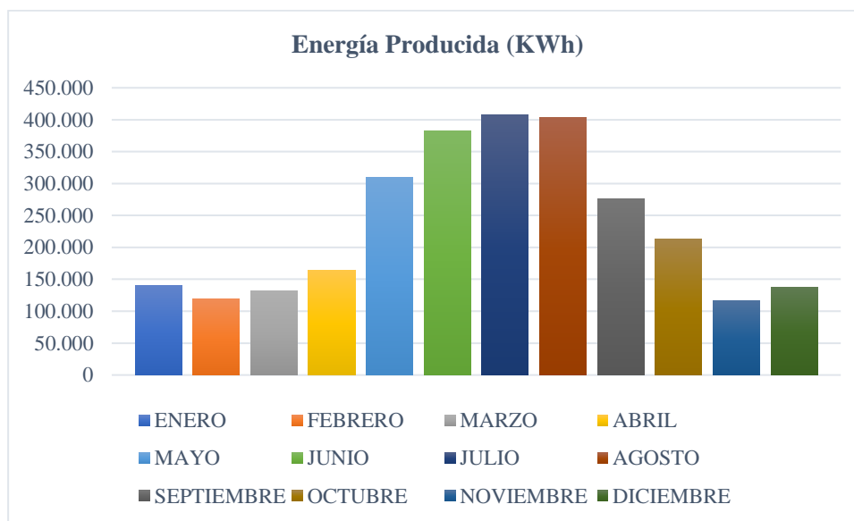
Figura 156. Energía producida mensual aerogenerador Nordex N60/1300.
