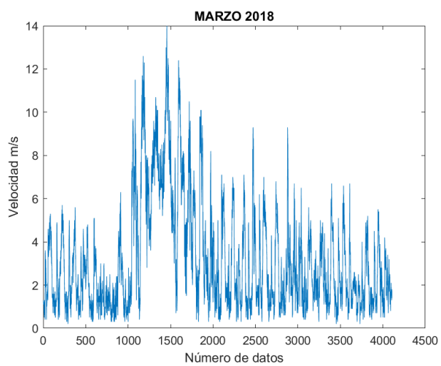
Figura 71. Velocidad del viento 03/2018.
