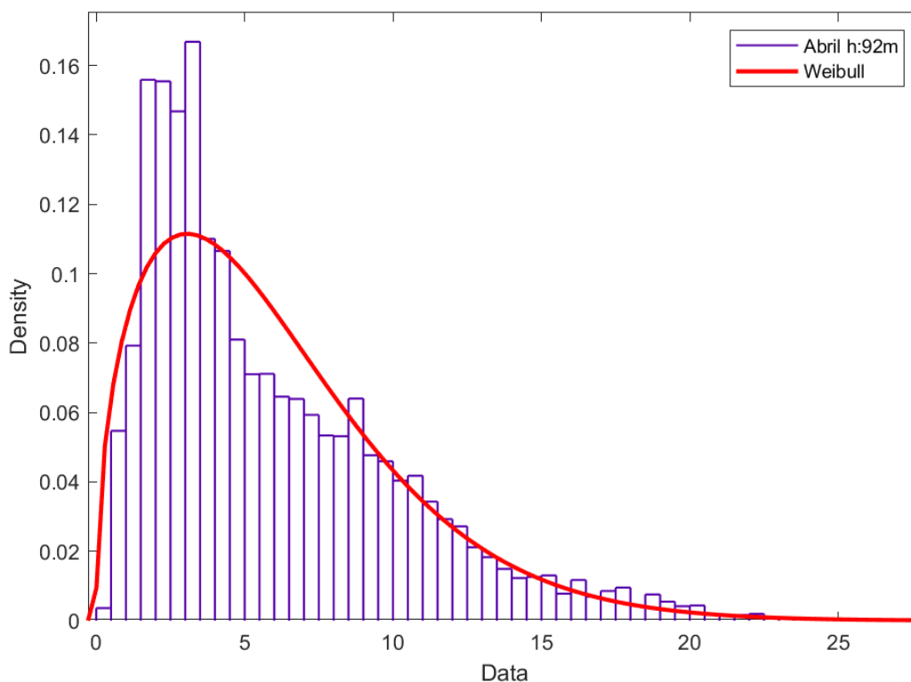
Figura 139. Distribución de Weibull mes abril H: 92 metros.
