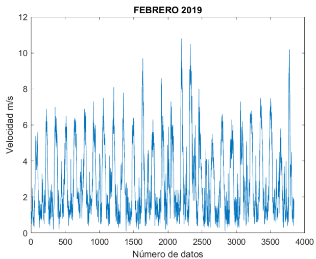
Figura 82. Velocidad del viento 02/2019.
