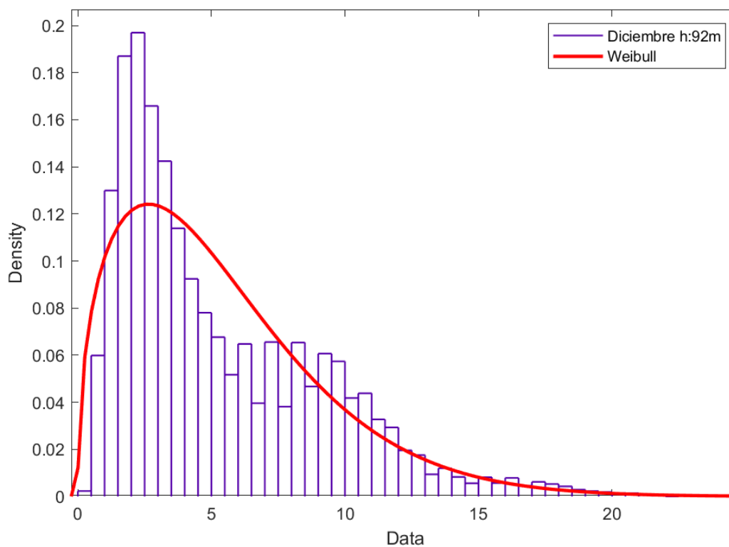
Figura 147. Distribución de Weibull mes diciembre H: 92 metros.
