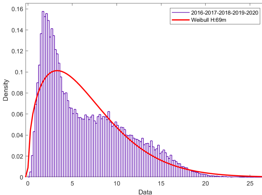
Figura 109. Distribución de Weibull muestra cinco años H: 69 metros.
