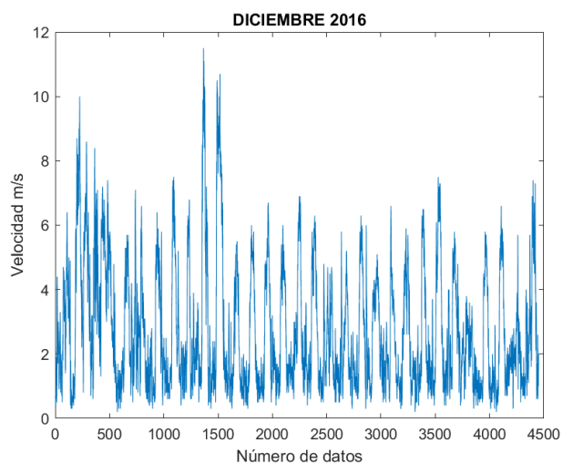
Figura 56. Velocidad del viento 12/2016.
