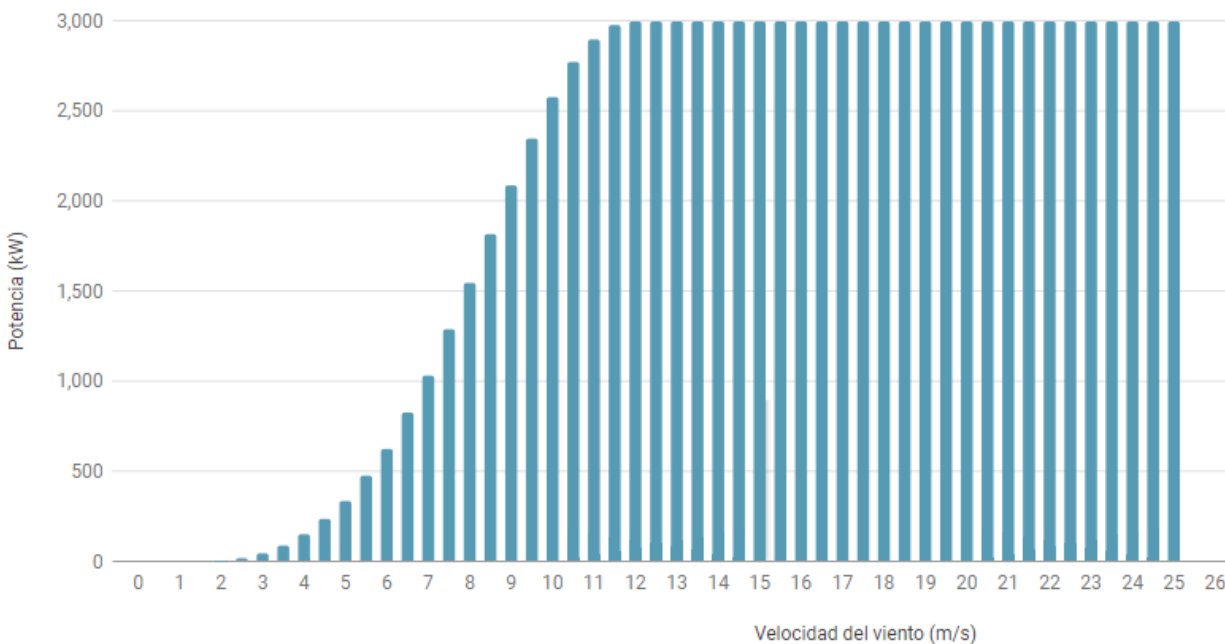
Figura 155. Curva de potencia aerogenerador Enercon E115/3000. Tomado de: ( The Wind Power, 2022 ).
