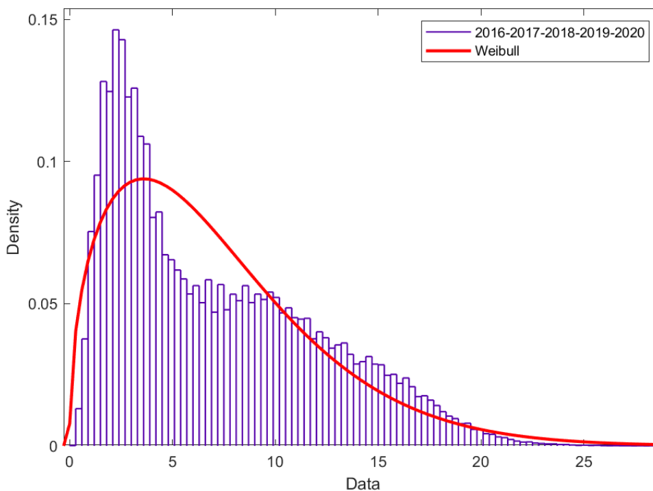
Figura 135. Distribución de Weibull muestra cinco años H: 92 metros.
