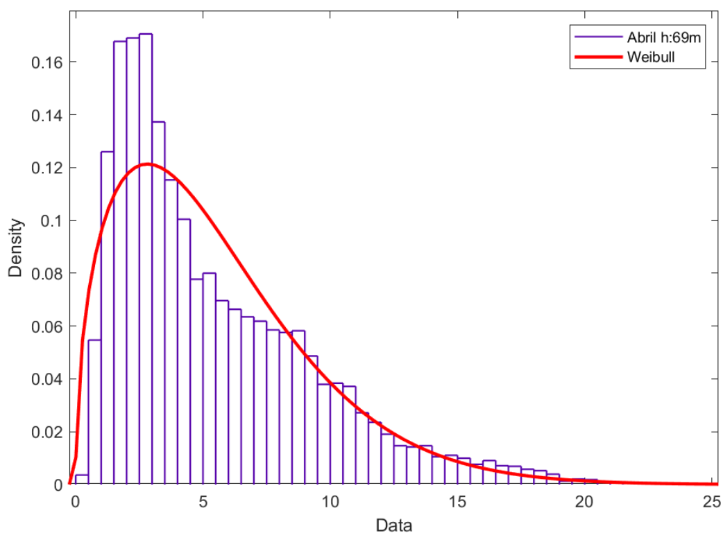
Figura 113. Distribución de Weibull mes abril H: 69 metros.
