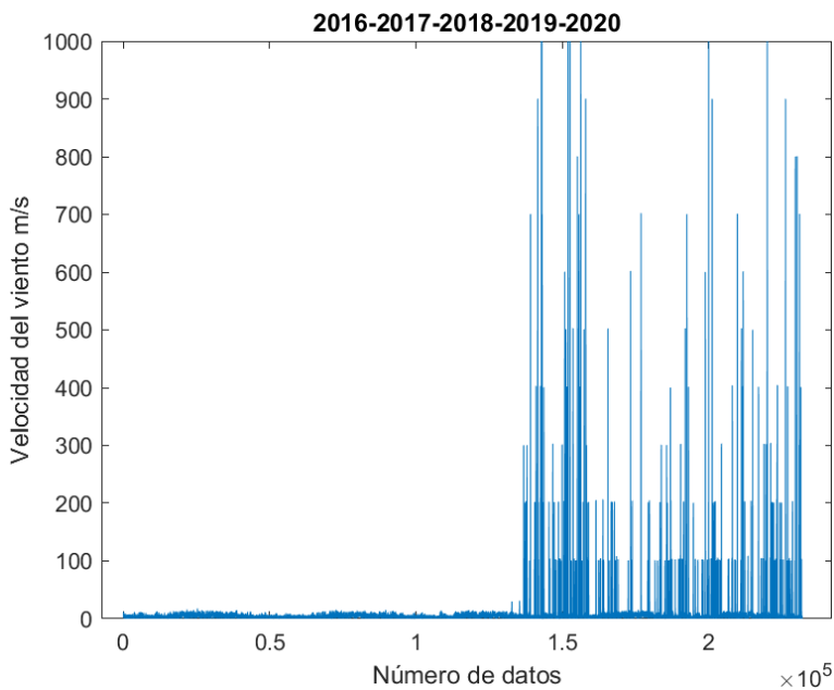
Figura 43. Velocidades del viento iniciales.
