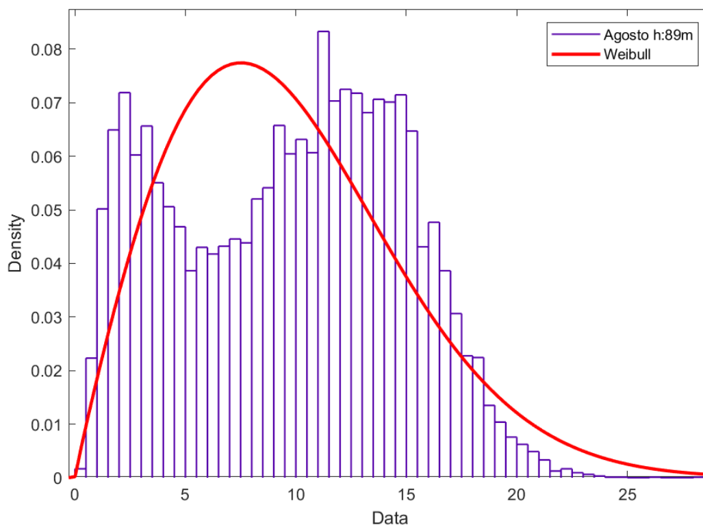
Figura 130. Distribución de Weibull mes agosto H: 89 metros.
