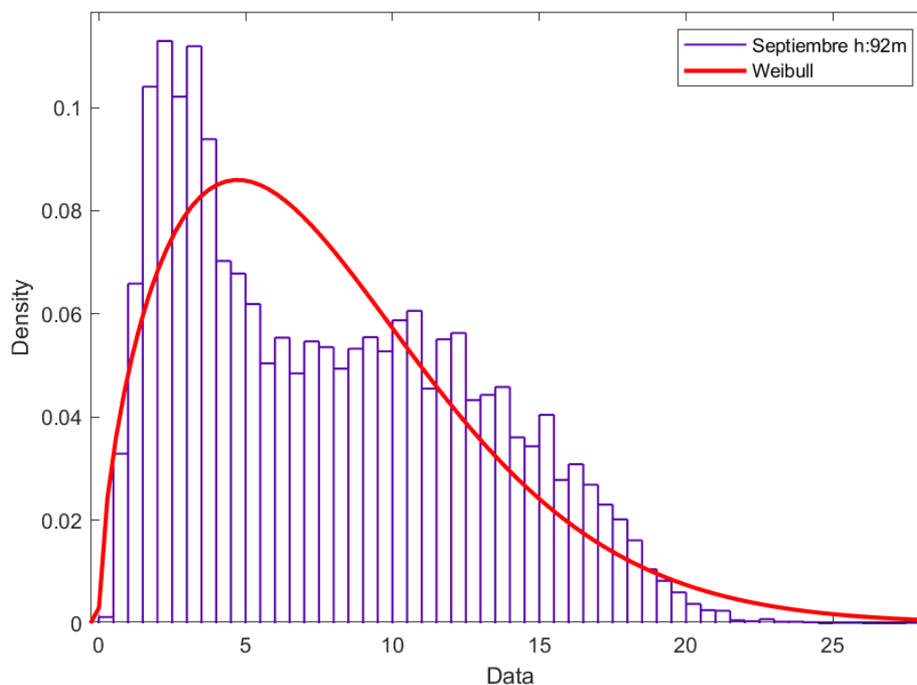
Figura 144. Distribución de Weibull mes septiembre H: 92 metros.
