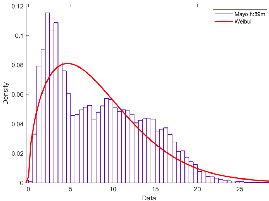
Figura 127. Distribución de Weibull mes mayo H: 89 metros.
