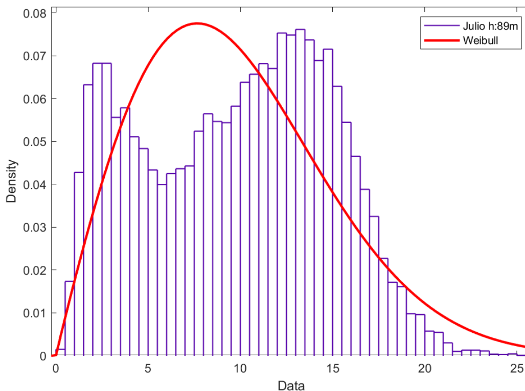
Figura 129. Distribución de Weibull mes julio H: 89 metros.
