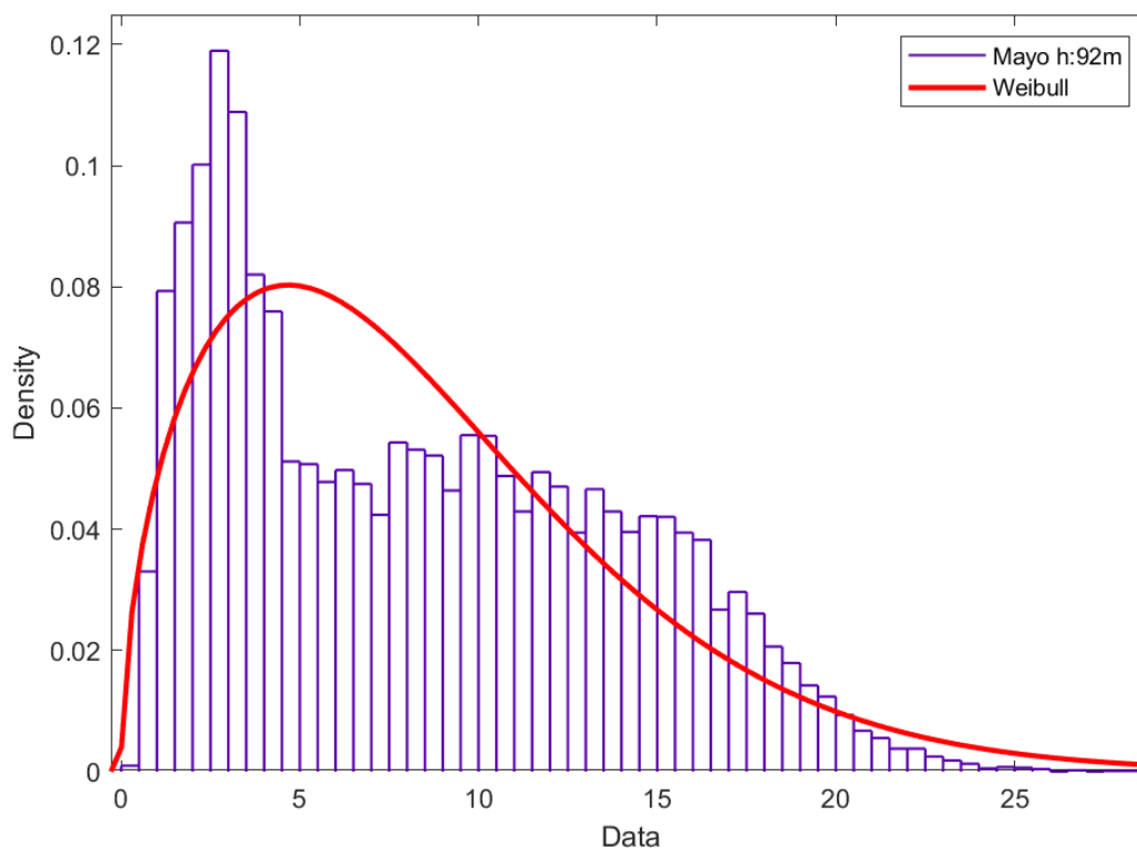
Figura 140. Distribución de Weibull mes mayo H: 92 metros.
