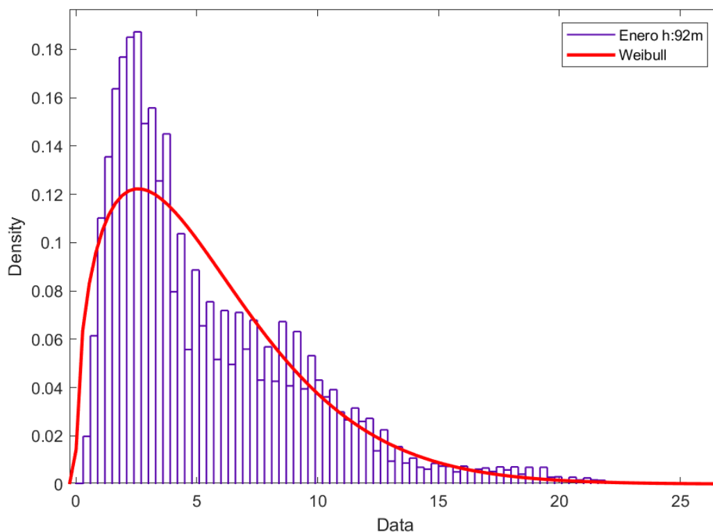
Figura 136. Distribución de Weibull mes enero H: 92 metros.
