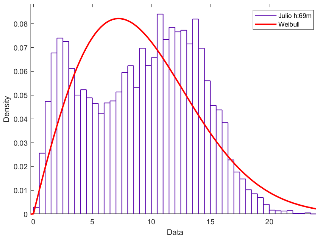
Figura 116. Distribución de Weibull mes julio H: 69 metros.
