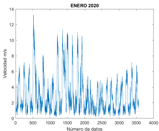
Figura 93. Velocidad del viento 01/2020.
