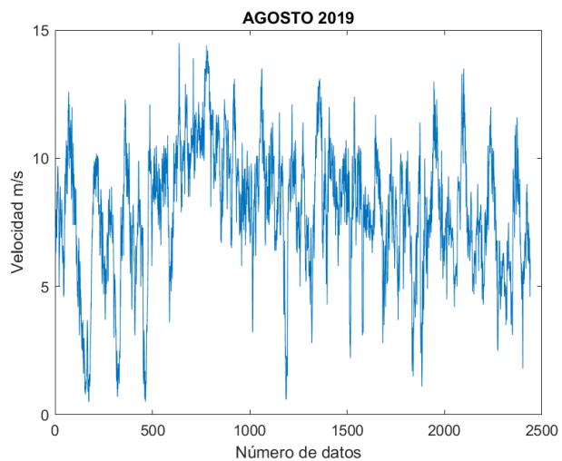
Figura 88. Velocidad del viento 08/2019.
