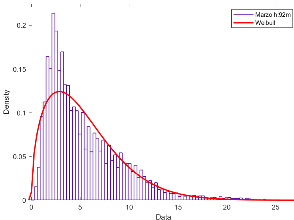
Figura 138. Distribución de Weibull mes marzo H: 92 metros.
