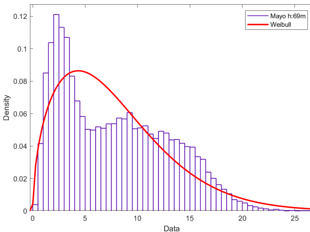
Figura 114. Distribución de Weibull mes mayo H: 69 metros.
