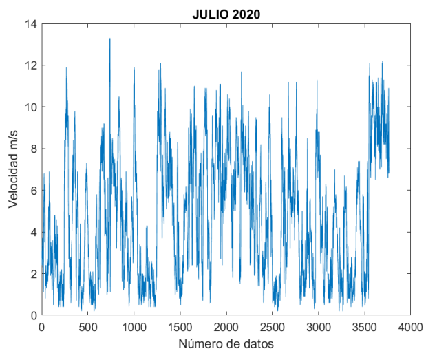
Figura 99. Velocidad del viento 07/2020.
