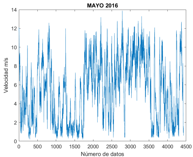
Figura 49. Velocidad del viento 05/2016.
