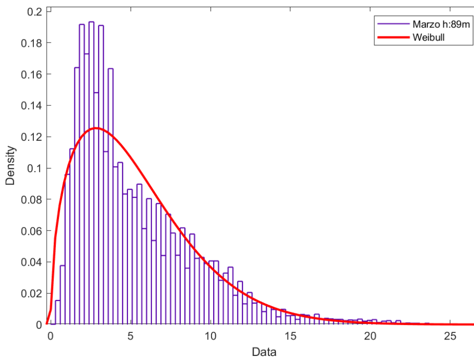
Figura 125. Distribución de Weibull mes marzo H: 89 metros.
