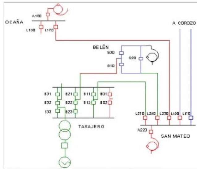
Figura 172. Anillo de tensión de 230 KV. Tomado de: Subestación eléctrica de San Mateo (Cácuta, 2012)
