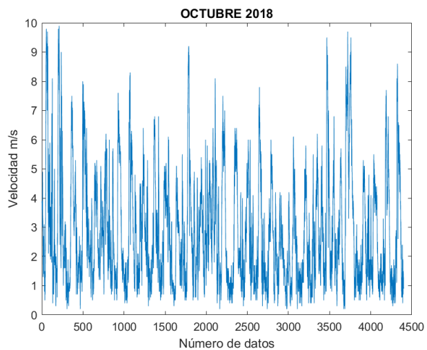
Figura 78. Velocidad del viento 10/2018.
