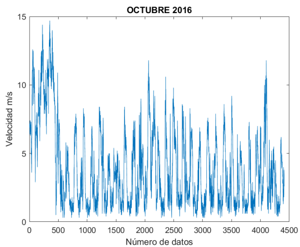
Figura 54. Velocidad del viento 10/2016.
