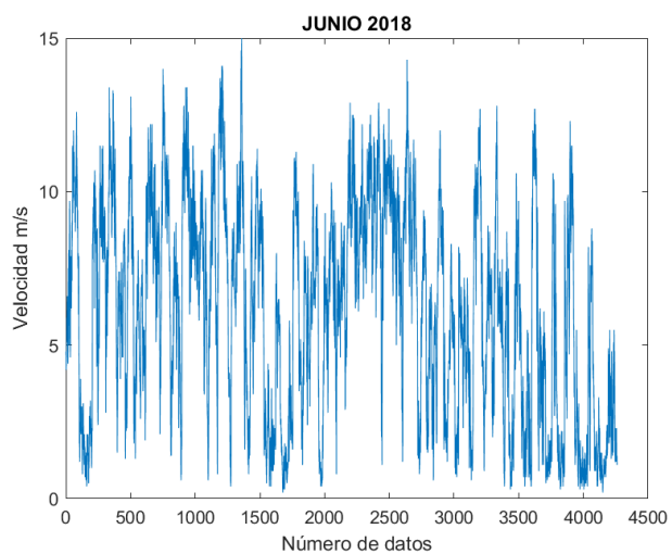
Figura 74. Velocidad del viento 06/2018.
