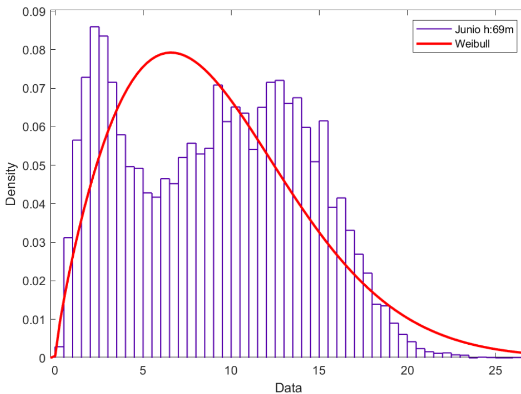
Figura 115. Distribución de Weibull mes junio H: 69 metros.
