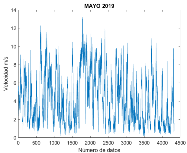
Figura 85. Velocidad del viento 05/2019.
