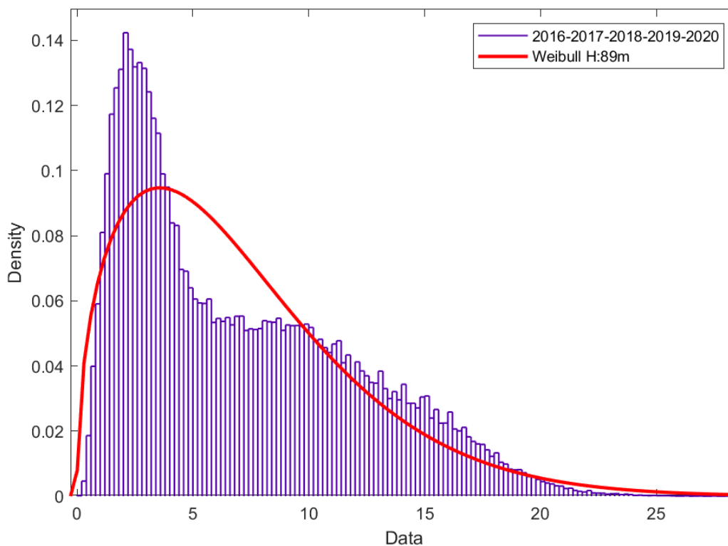
Figura 122. Distribución de Weibull muestra cinco años H: 89 metros.
