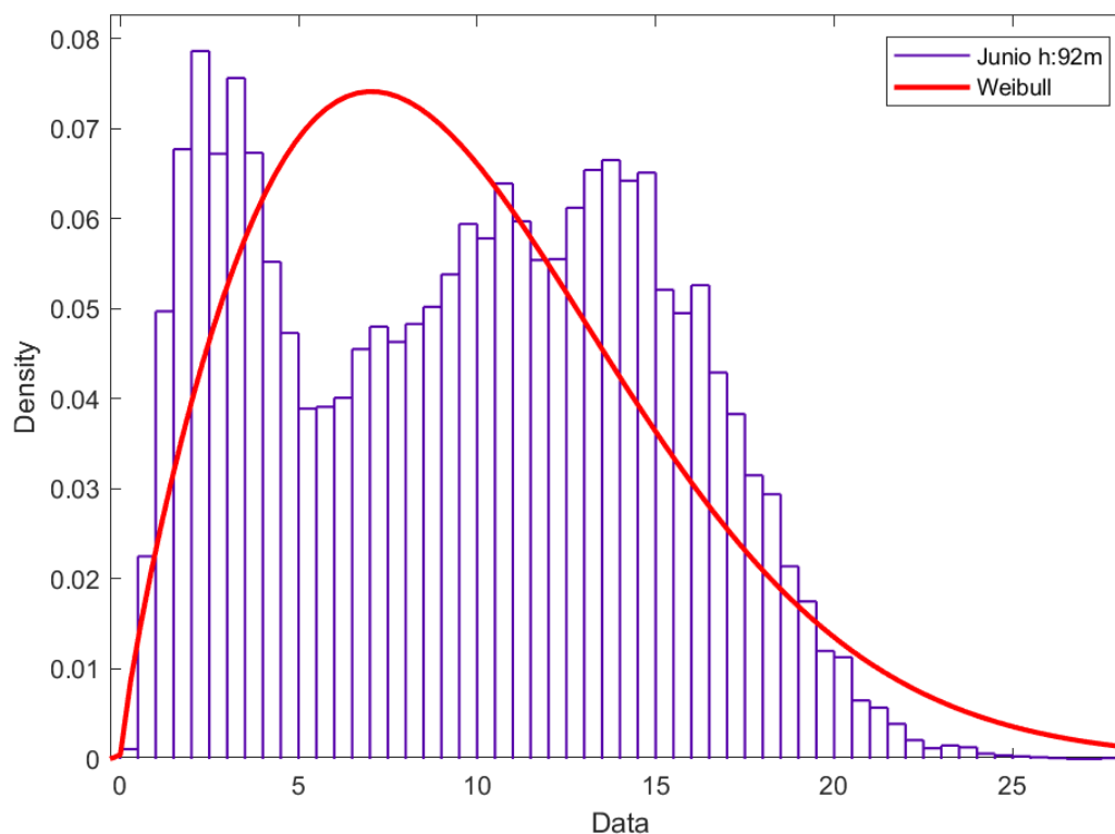
Figura 141. Distribución de Weibull mes junio H: 92 metros.
