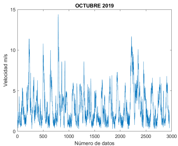
Figura 90. Velocidad del viento 10/2019.
