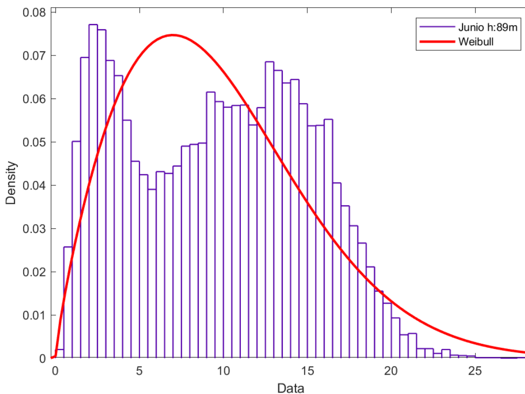
Figura 128. Distribución de Weibull mes junio H: 89 metros.
