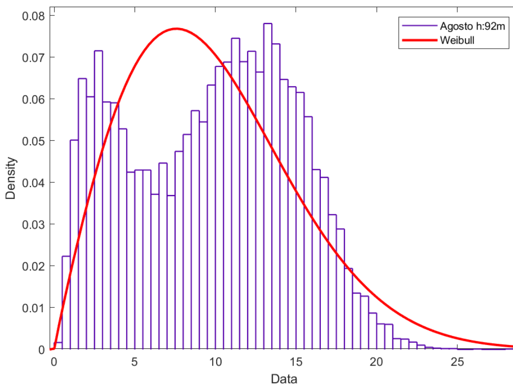
Figura 143. Distribución de Weibull mes agosto H: 92 metros.
