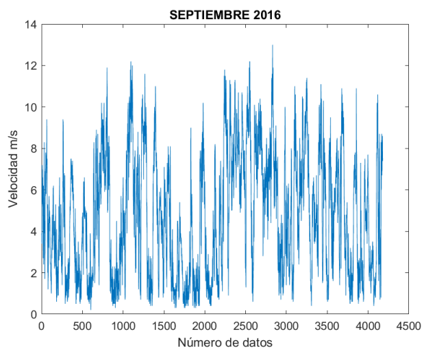
Figura 53. Velocidad del viento 09/2016.
