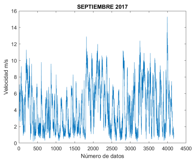
Figura 65. Velocidad del viento 09/2017.
