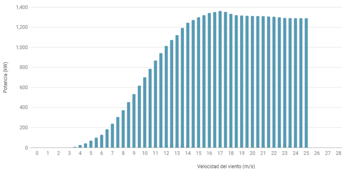
Figura 149. Curva de potencia aerogenerador Nordex N60/1300. Tomado de: ( The Wind Power , 2022).
