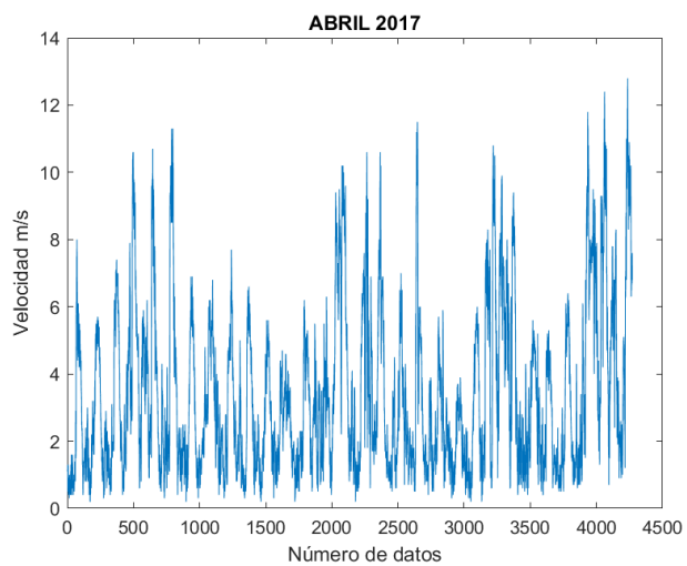
Figura 60. Velocidad del viento 04/2017.
