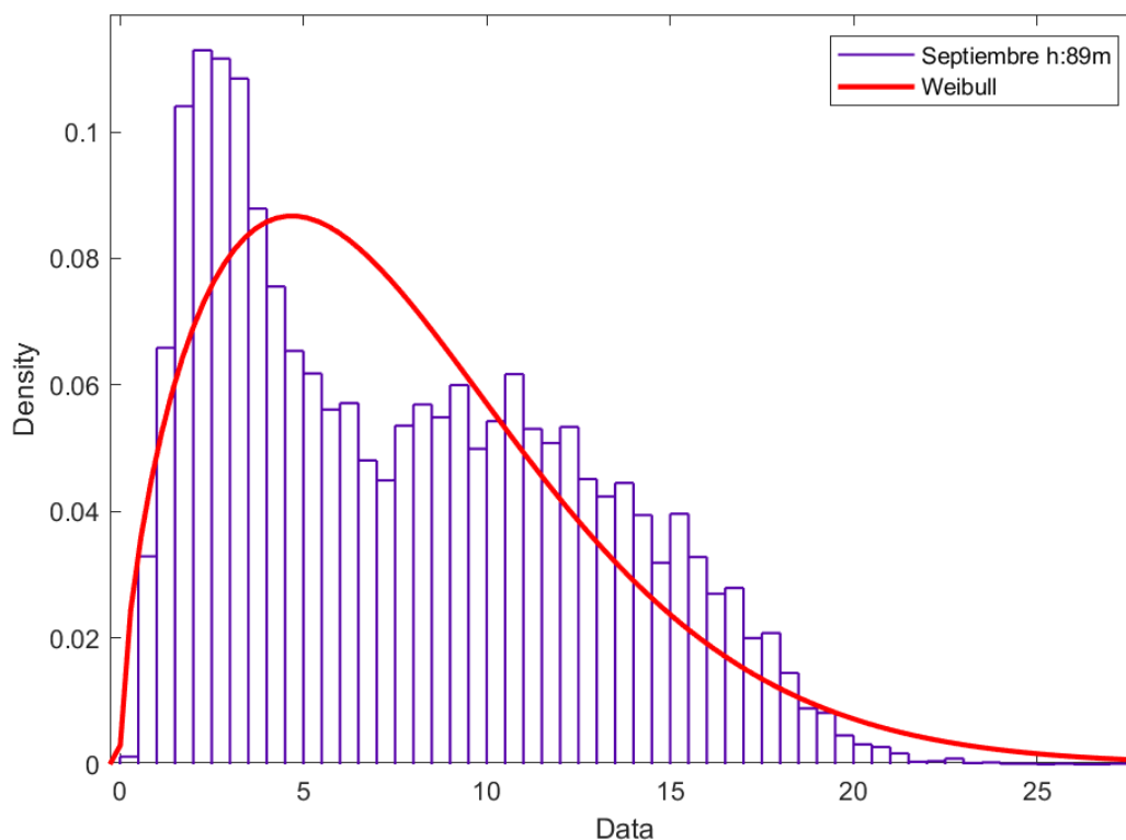
Figura 131. Distribución de Weibull mes septiembre H: 89 metros.
