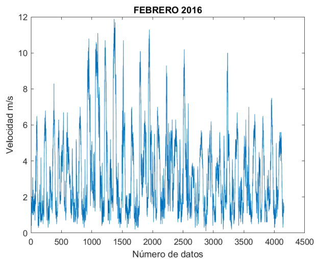
Figura 46. Velocidad del viento 02/2016.
