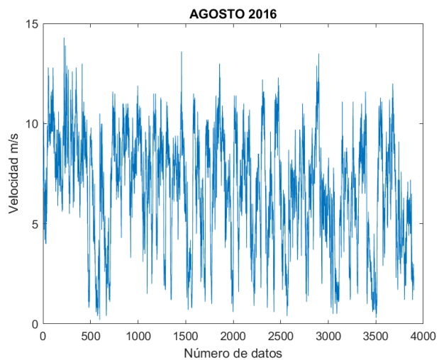
Figura 52. Velocidad del viento 08/2016.
