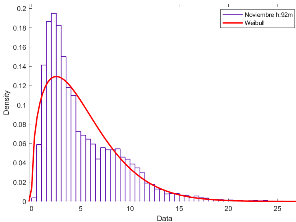
Figura 146. Distribución de Weibull mes noviembre H: 92 metros.
