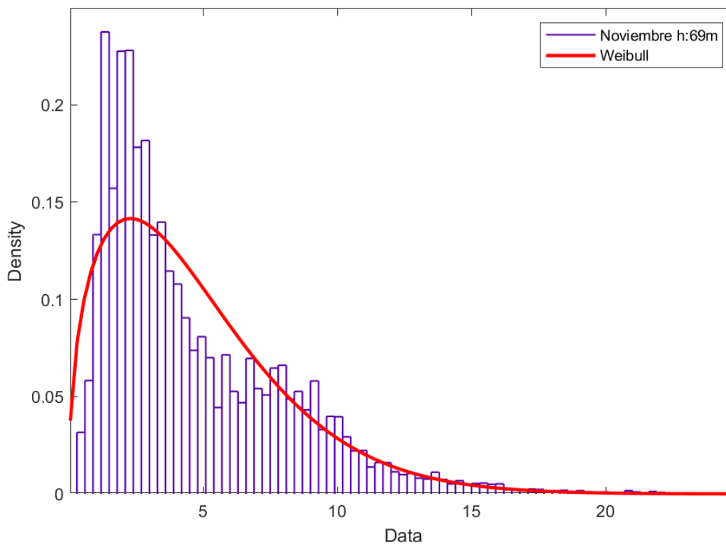
Figura 120. Distribución de Weibull mes noviembre H: 69 metros.
