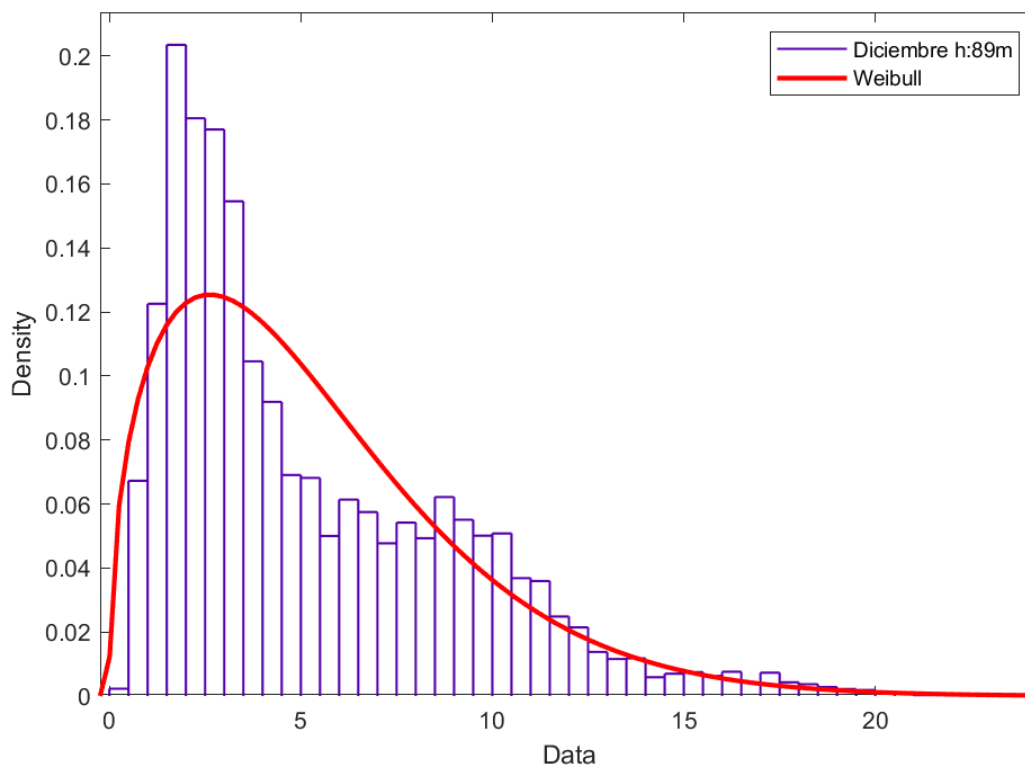
Figura 134. Distribución de Weibull mes diciembre H: 89 metros.
