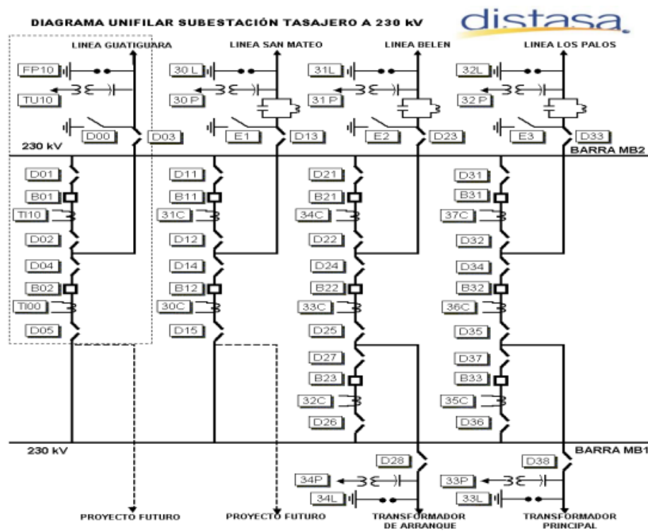
Figura 182. Diagrama unifilar subestación Tasajero. Tomado de: (DISTASA S.A, 2017).
