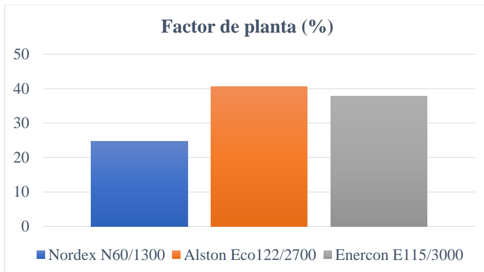
Figura 161. Factor de planta 1 año.
