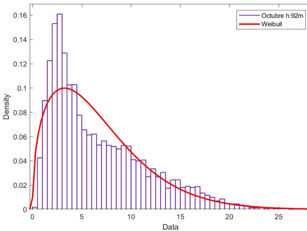
Figura 145. Distribución de Weibull mes octubre H: 92 metros.
