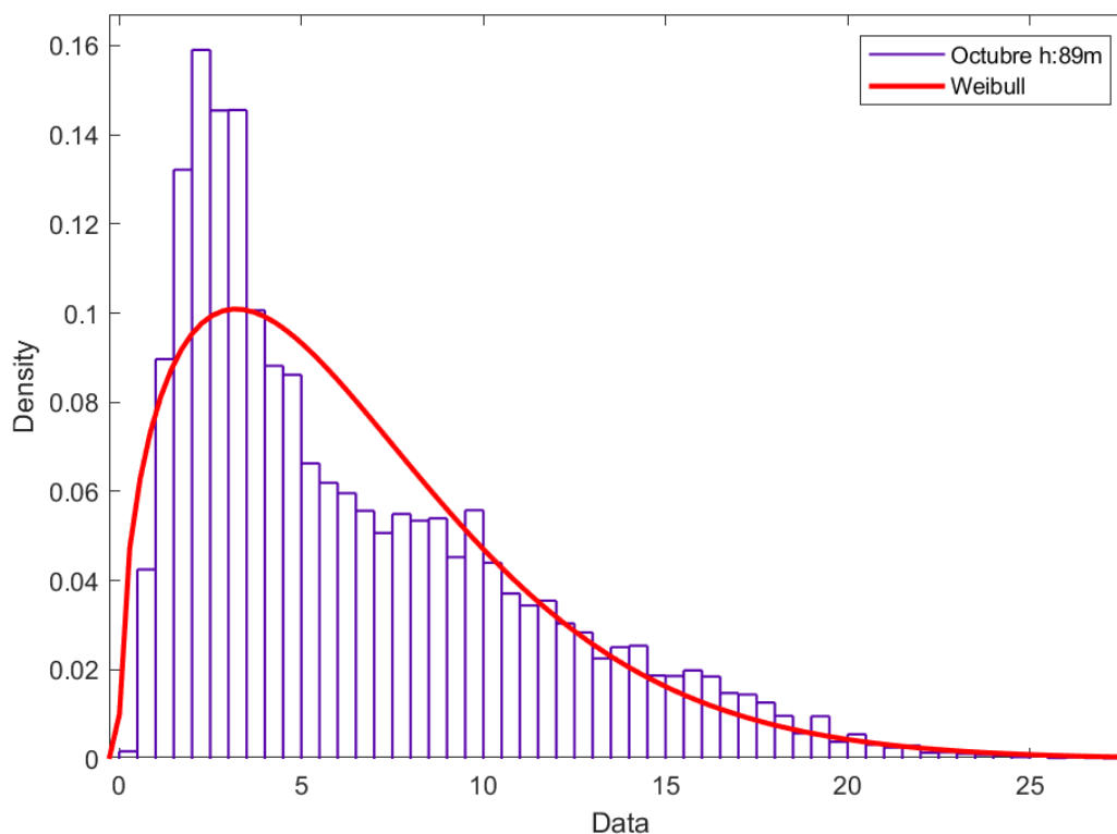
Figura 132. Distribución de Weibull mes octubre H: 89 metros.
