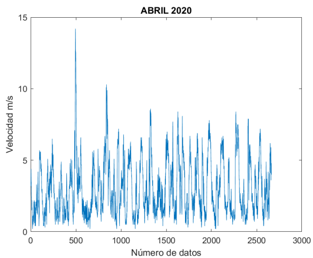
Figura 96. Velocidad del viento 04/2020.
