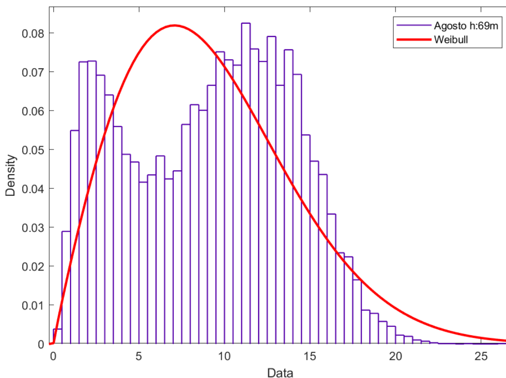
Figura 117. Distribución de Weibull mes agosto H: 69 metros.
