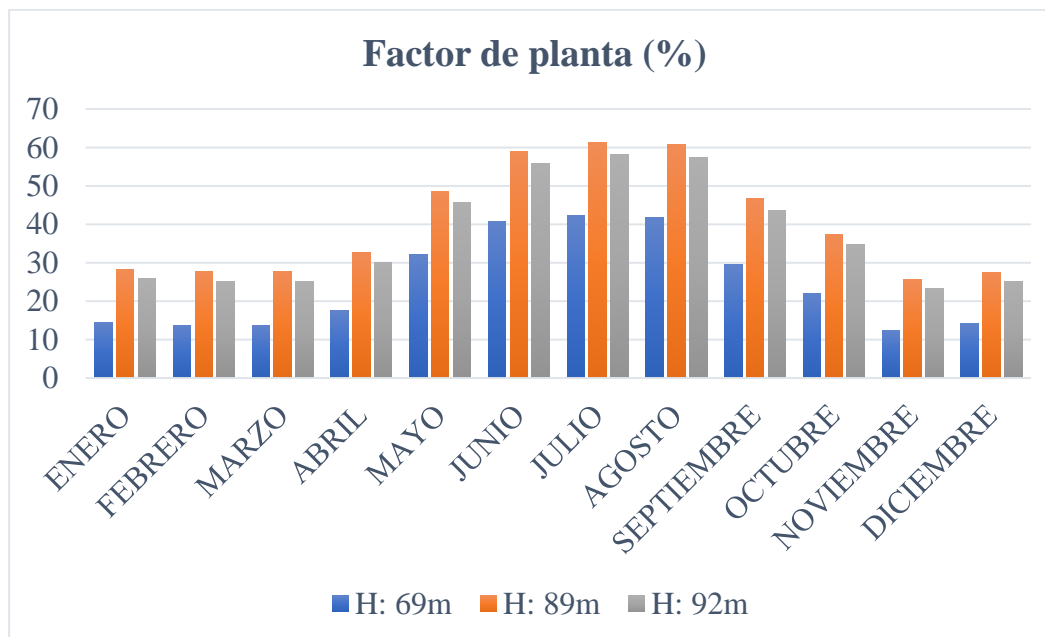
Figura 162. Factor de planta mensual.
