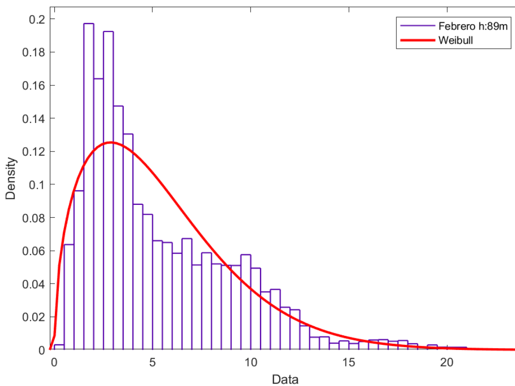
Figura 124. Distribución de Weibull mes febrero H: 89 metros.
