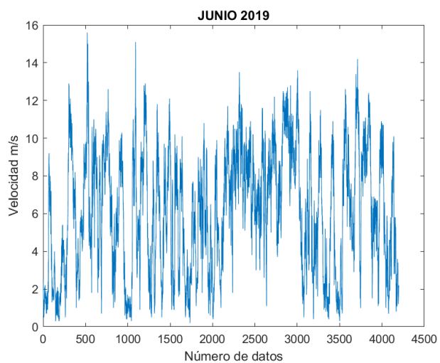
Figura 86. Velocidad del viento 06/2019.
