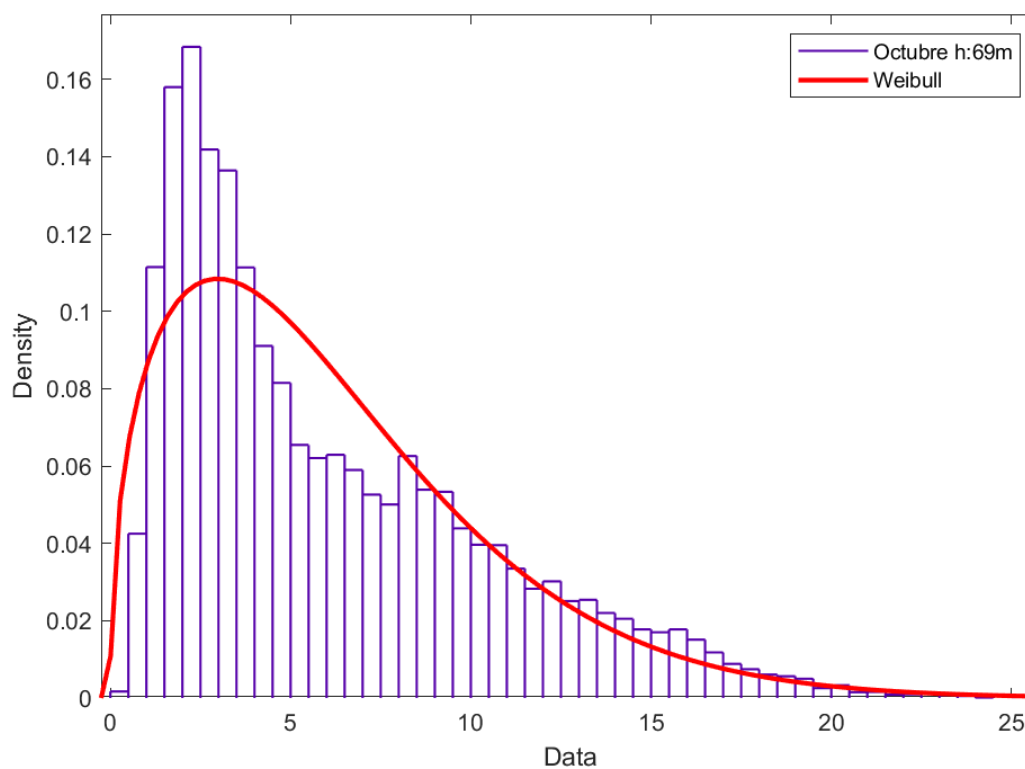
Figura 119. Distribución de Weibull mes octubre H: 69 metros.
