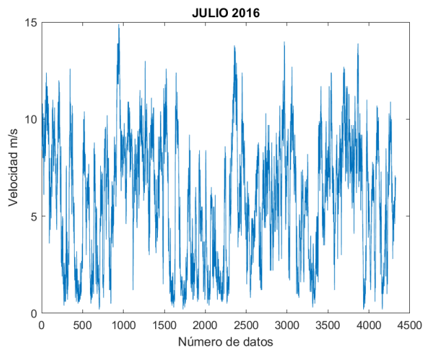
Figura 51. Velocidad del viento 07/2016.
