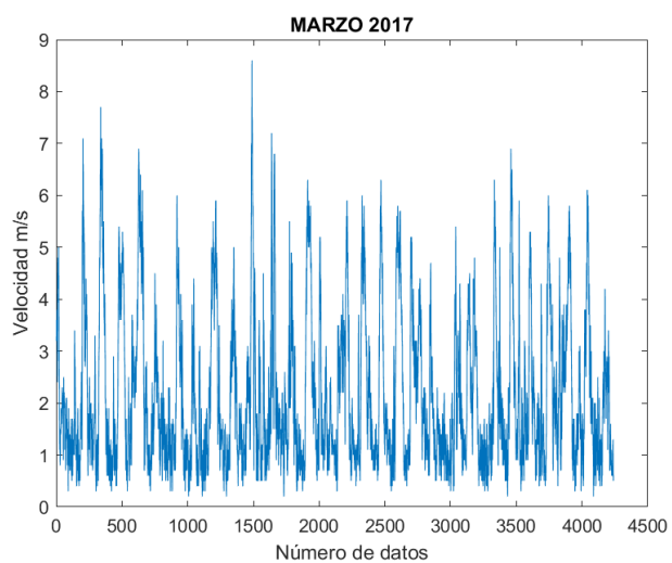
Figura 59. Velocidad del viento 03/2017.
