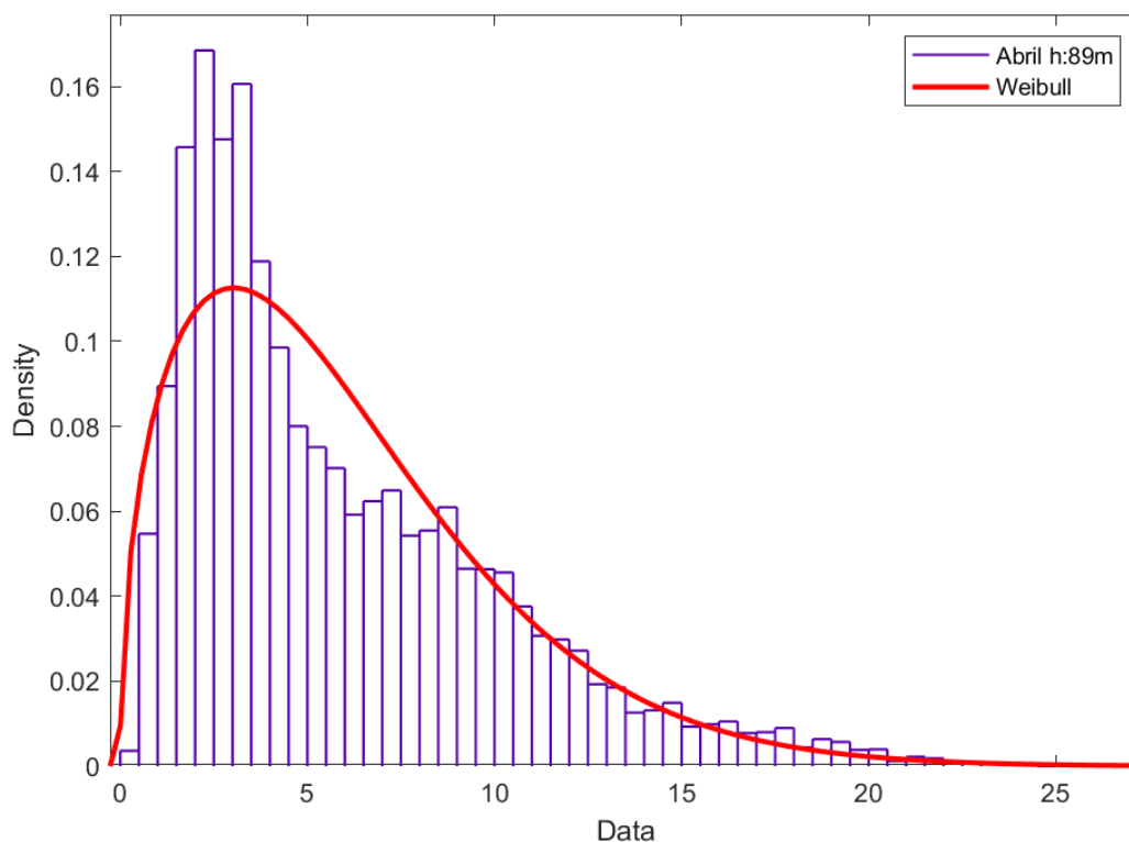
Figura 126. Distribución de Weibull mes abril H: 89 metros.
