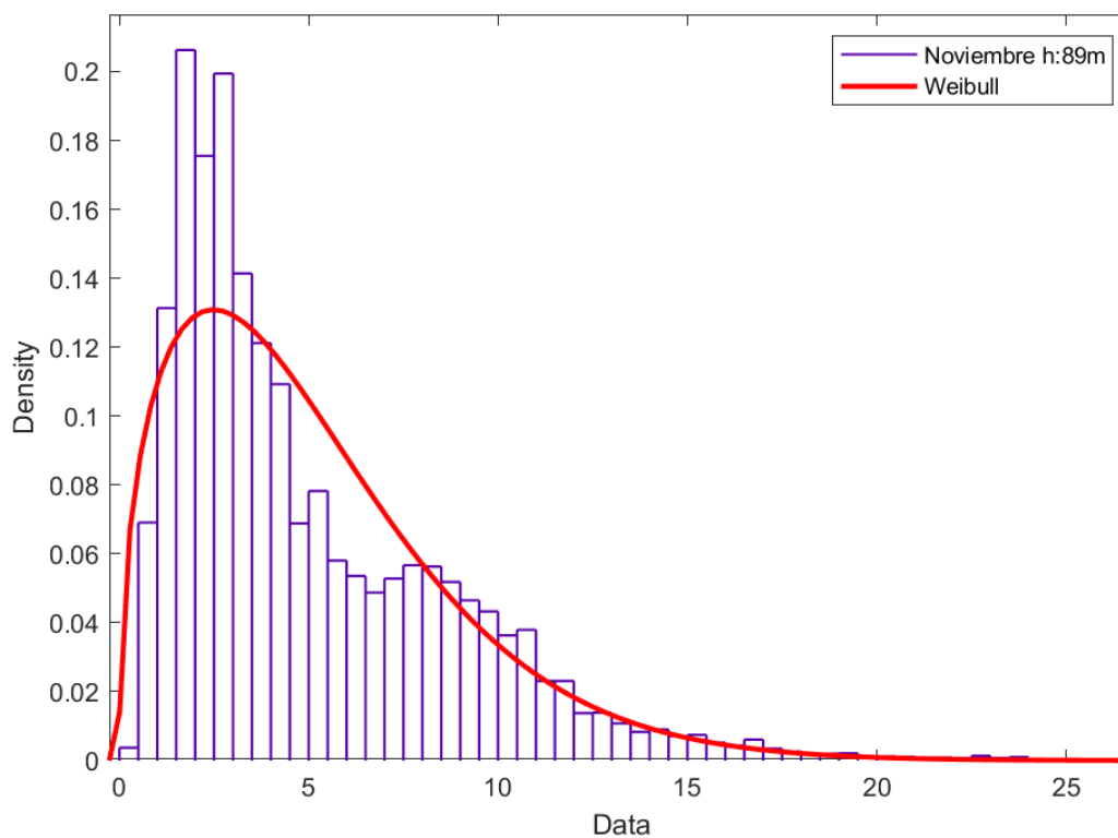
Figura 133. Distribución de Weibull mes noviembre H: 89 metros.
