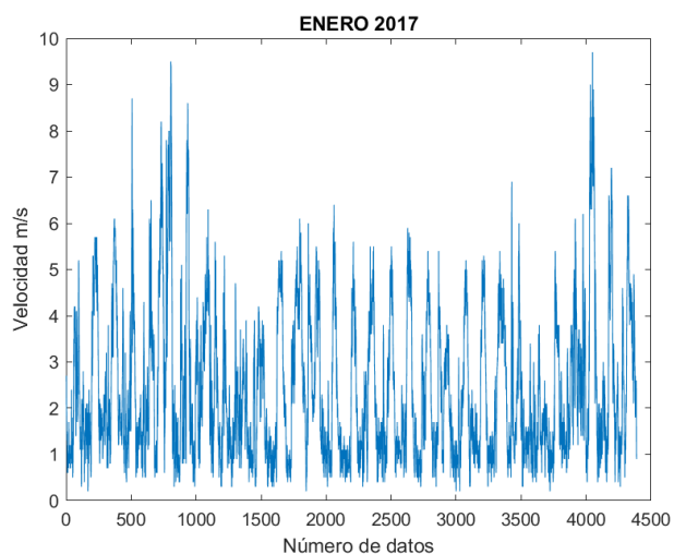
Figura 57. Velocidad del viento 01/2017.
