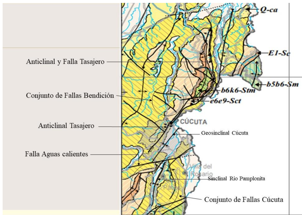
Figura 166. Estructuras geológicas – Cúcuta – Cerro Tasajero. Fuente: Atlas geológico de Colombia ( Servicio Geológico Colombiano, 2015 ).
