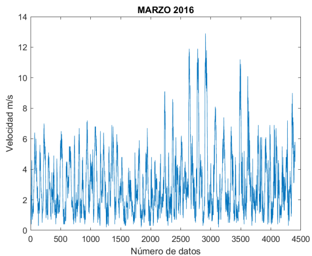
Figura 47. Velocidad del viento 03/2016.
