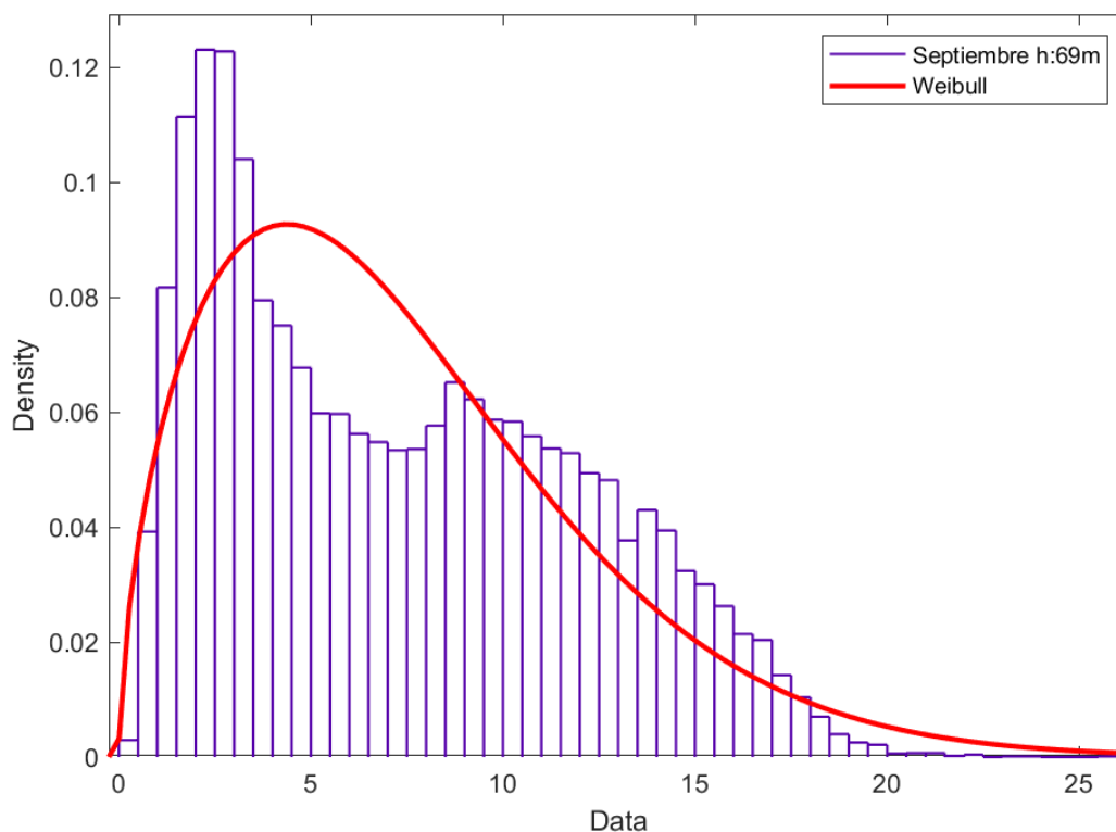
Figura 118. Distribución de Weibull mes septiembre H: 69 metros.
