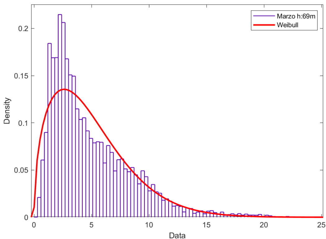
Figura 112. Distribución de Weibull mes marzo H: 69 metros.
