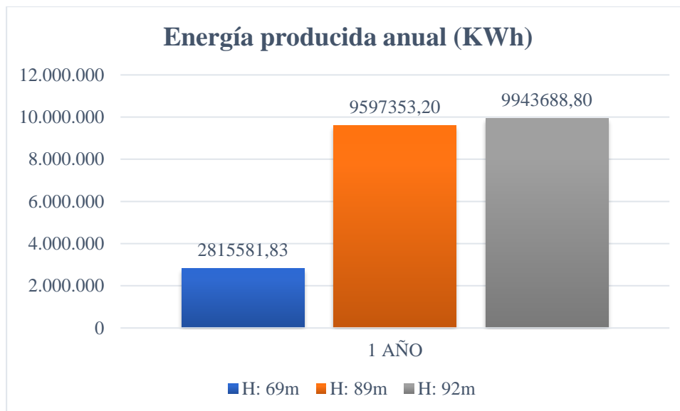
Figura 159. Energía producida anual.
