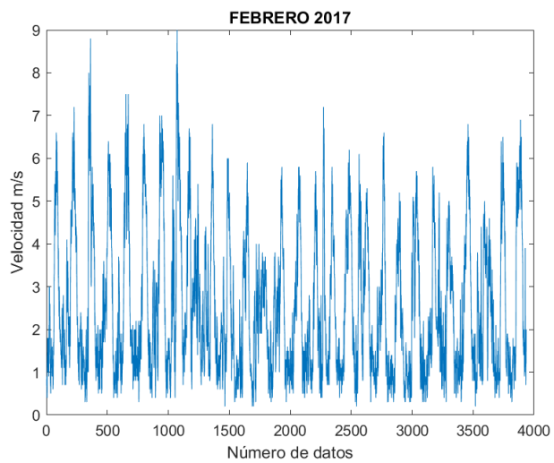
Figura 58. Velocidad del viento 02/2017.
