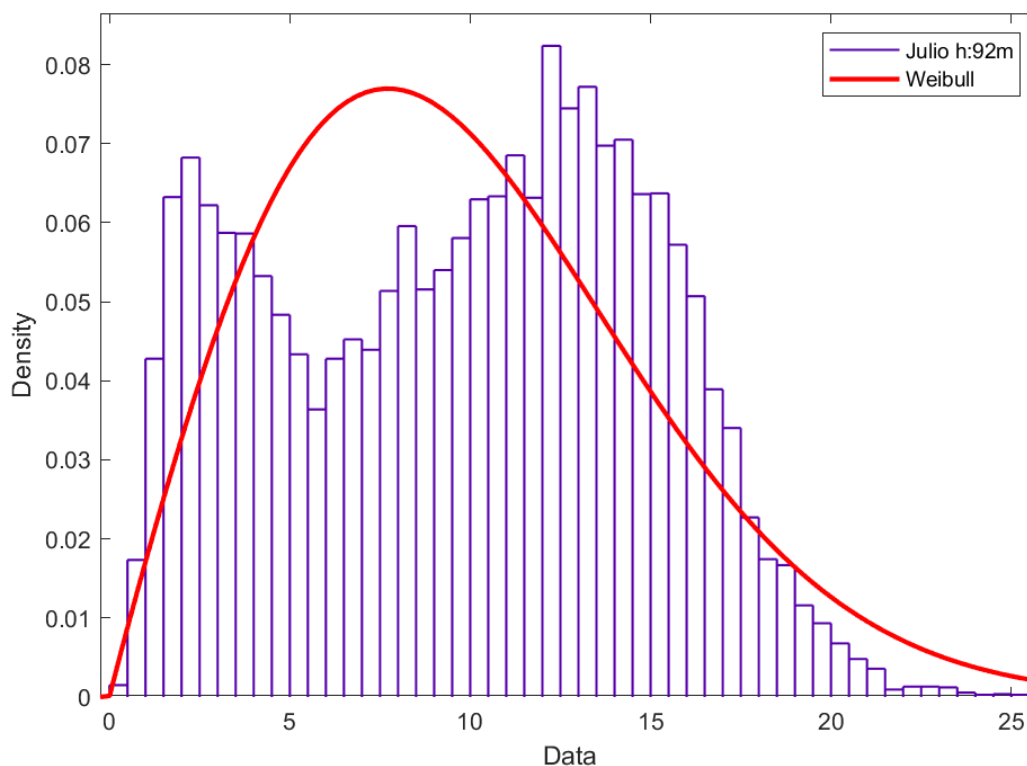
Figura 142. Distribución de Weibull mes julio H: 92 metros.
